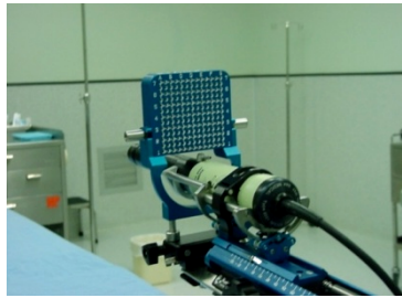
Hình 3. Hệ thống giá đỡ và ma trận
