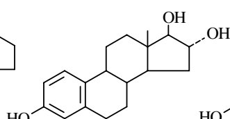
Estriol
