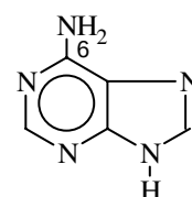
Adenin
