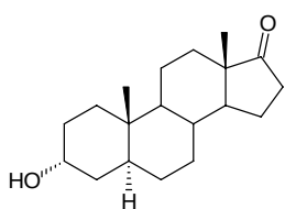
Androsteron
