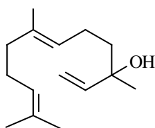
Nerolidol
