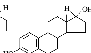
β-Estradiol (Estradiol-17α)
