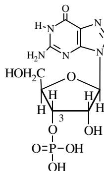
Guanylic
