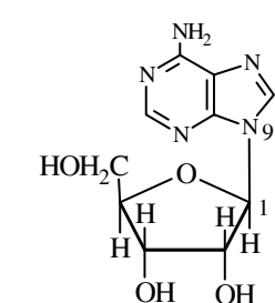
Adenosin ( Ribose + Adenin )
