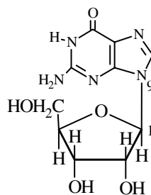
Guanosin ( Ribose + Guanin )
