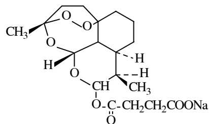
Natri artesunat
