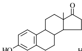
Estron
