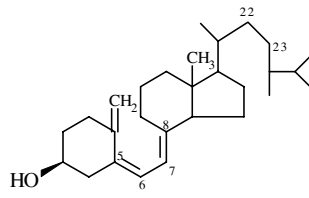
Vitamin D 4
