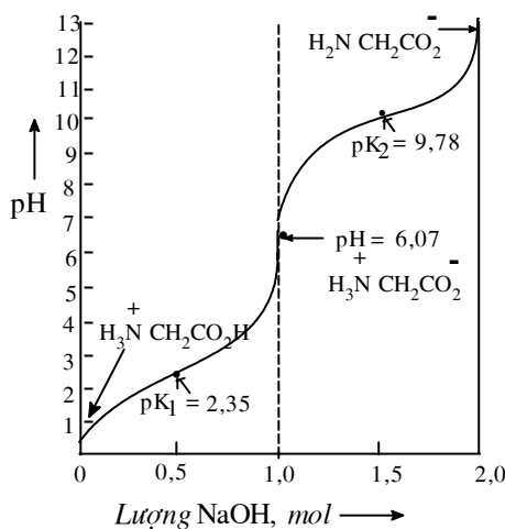
Đường cong chuẩn độ \text{NH}_3^+\text{CH}_2\text{COOH}
