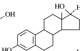
α-Estradiol (Estradiol-17β)
