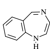
1,4-Benzodiazepin
