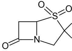
Sulbactam
