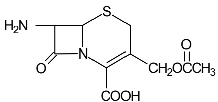
7-ACA
