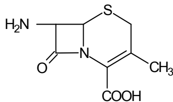
7-ADCA
