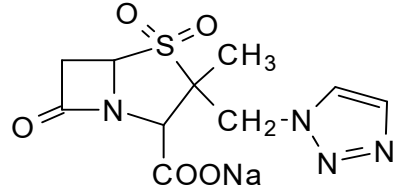
Tazobactam
