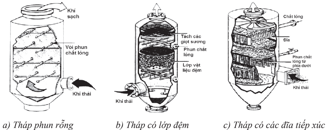
Hình 4. Các loại tháp rửa khí
