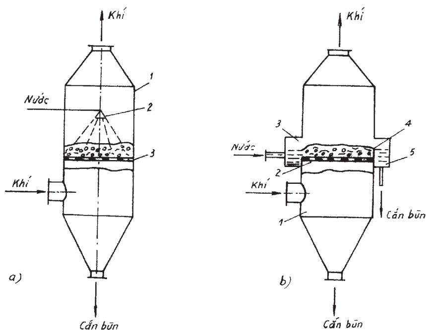
a) Loại giội nước dập khí 1 - vỏ thiết bị; 2 - vòi phun; 3 - đĩa đục lỗ
