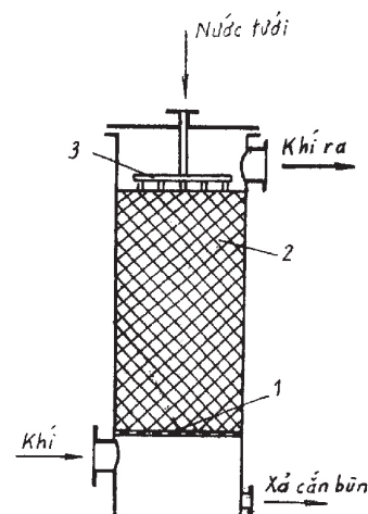
b) Tháp rửa khí có lớp đệm
