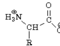
Dạng zwitterion chủ yếu trong dung dịch
