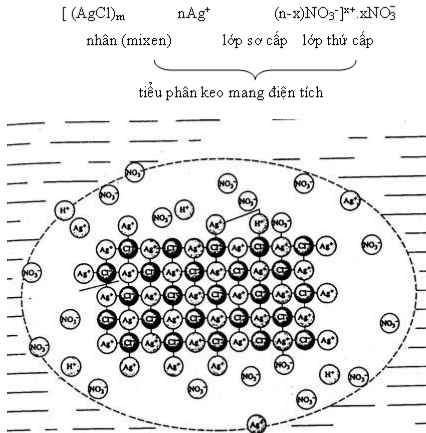
Hình 9.6. Cấu tạo hạt keo AgCl trong dung dịch AgNO 3
