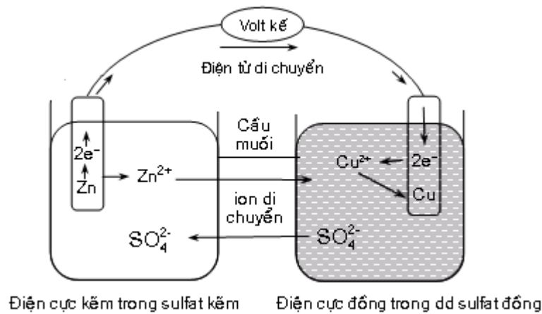
Hình 8.4. Sơ đồ cấu tạo 1 pin điện hoá
