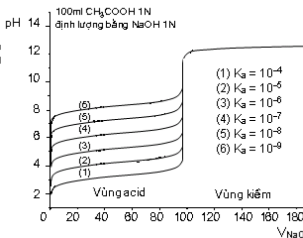
Hình 7.19. Trung hoà các acid yếu (1N) có K a khác nhau bằng base mạnh (c)
