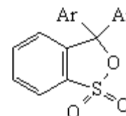
Hình 7.9. Sulfon phtalein
