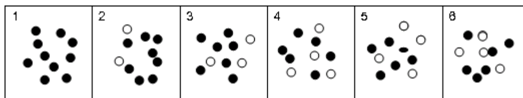
Hình 2.1. Chuyển 2\text{NO}_2 (\text{k}) \rightleftharpoons \text{N}_2\text{O}_4 (\text{k}) , hệ thống cân bằng ở các ô 4, 5 và 6
